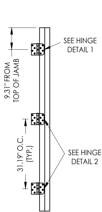
HINGE JAMB
